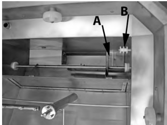
Imagen 27 Tamiz del fondo y sensor de nivel
