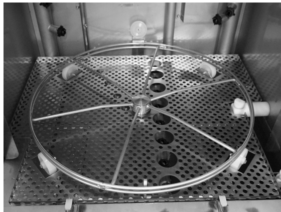
Fig. 35 Kosárkerék
