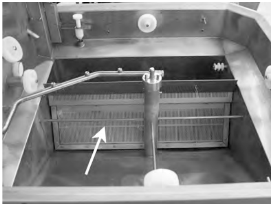
Bild 26 Granuldämpare
