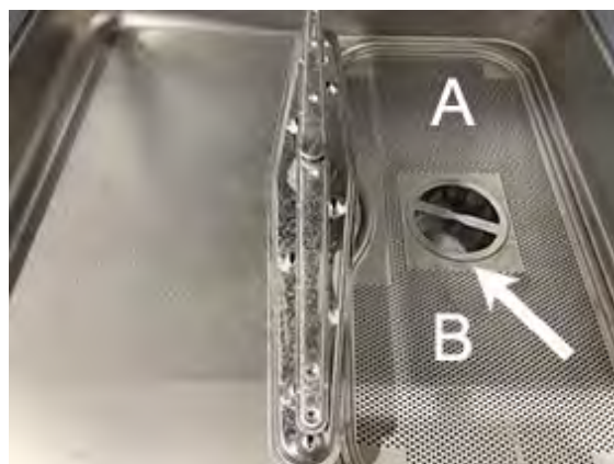
Figura 15 Rimuovere le griglie della vasca e il filtro
