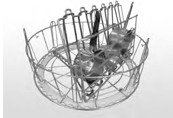
Abbildung 20 Multiflex-Halter
