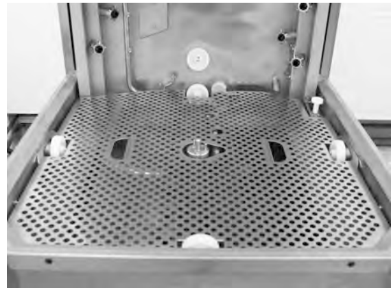
Abbildung 28 Tankgitter
