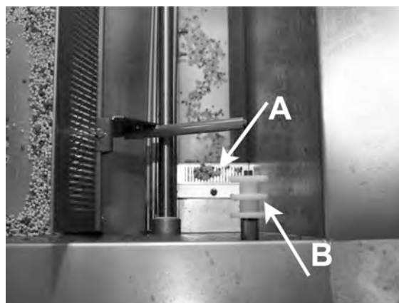
εικόνα 29 Καθαρίστε τη σήτα πυθμένα και τον αισθητήρα στάθμης
