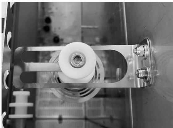
Abbildung 40 Überlaufarmatur
