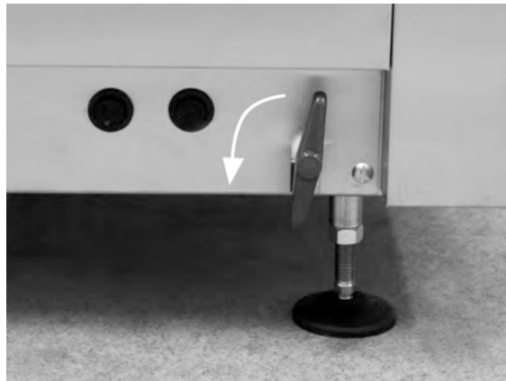
εικόνα 6 Άνοιγμα της βαλβίδας αποστράγγισης
