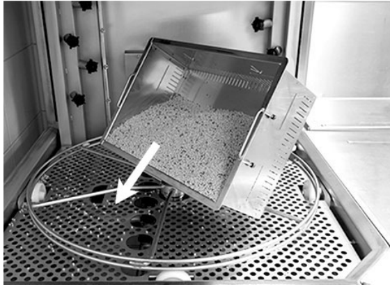
Bild 5 Granulutfyllning
