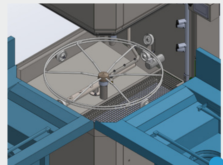
Abb. 4 Eckanordnung mit Fronttisch und Beistelltisch
