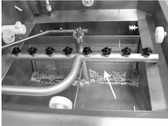
Kuva 28 Raesiivilän puhdistaminen
